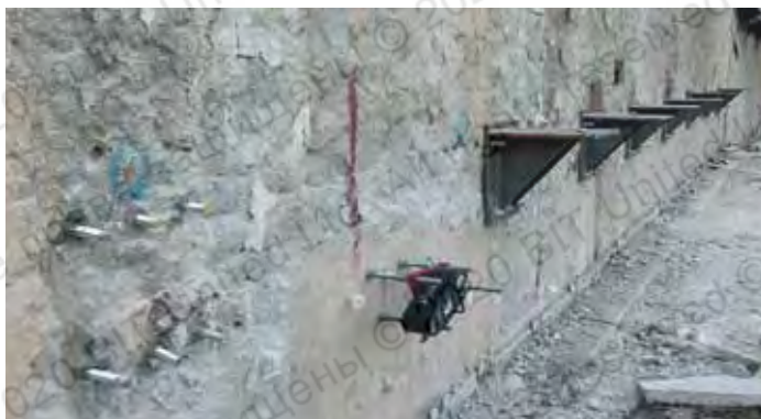
Установка опорных столиков для монтажа распорной системы ограждения котлована (Павелецкая площадь, г. Москва, 2018 г.)
